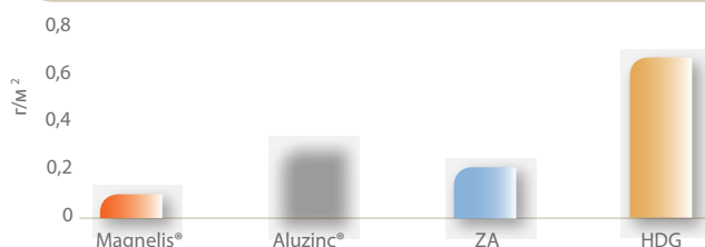
Убыль веса в агрессивных средах
