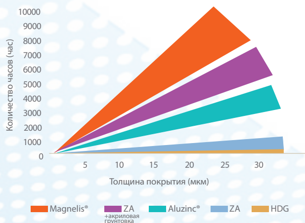
Количество часов до появления 5% красной ржавчины
