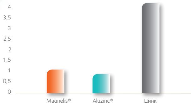
Снижение массы цинка (г/м²/год)
